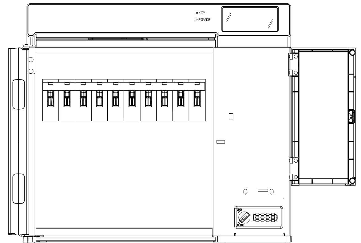
開扉状態
