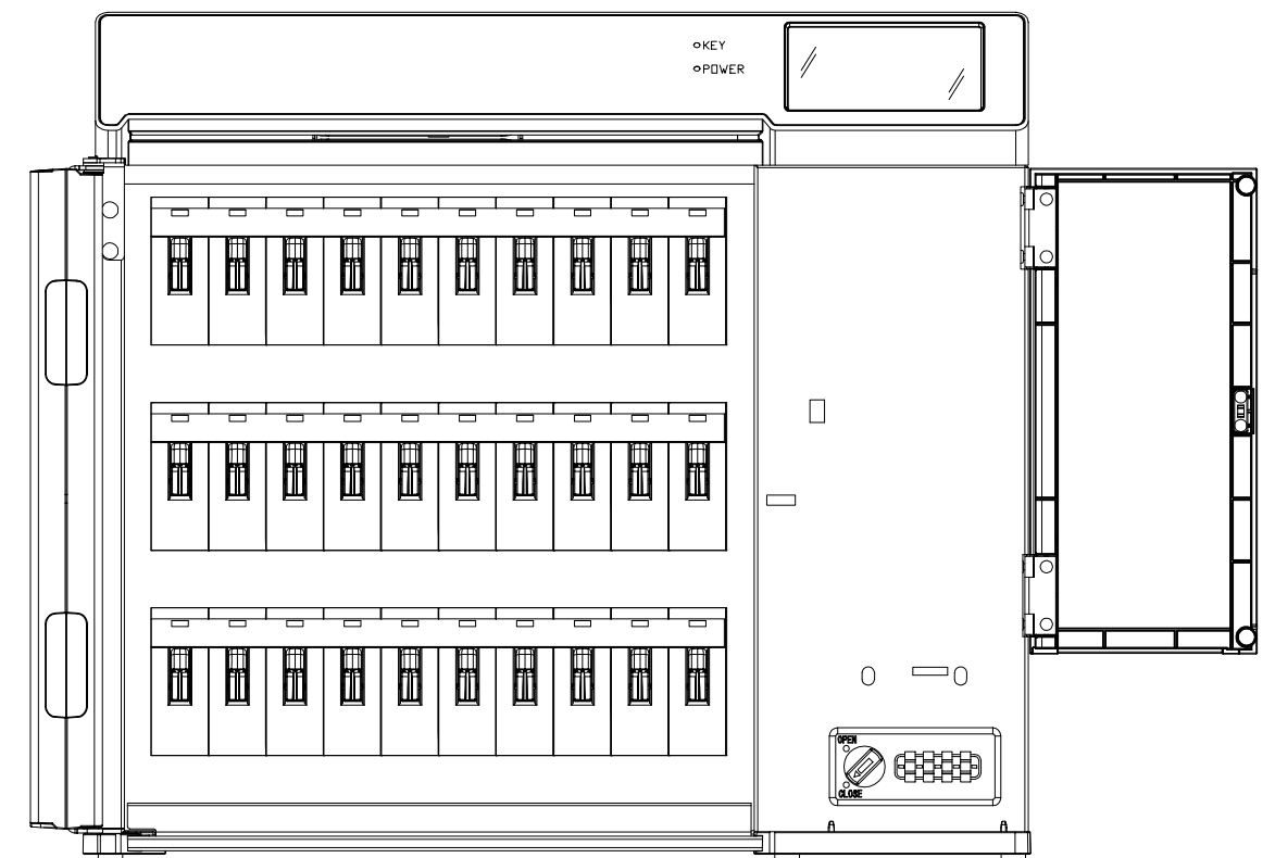
開扉状態
