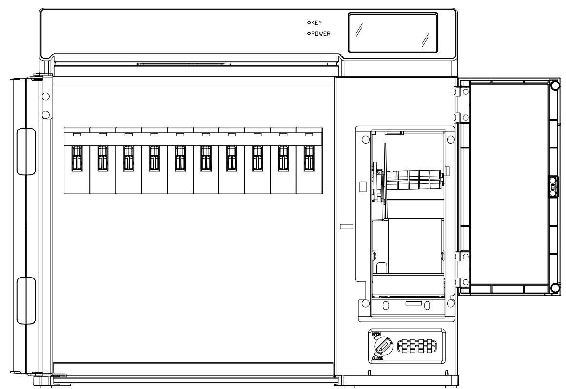
開扉状態
