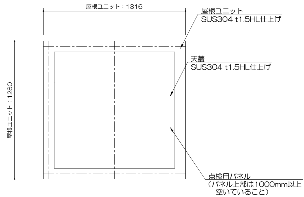
屋根伏図
